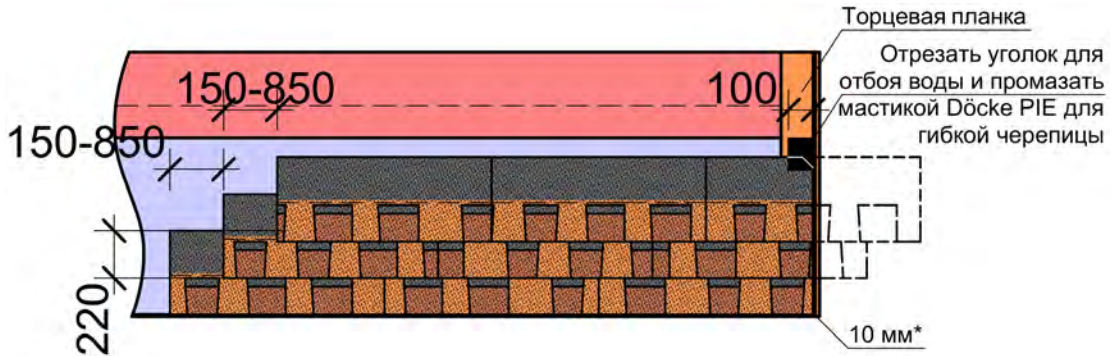
Рис. 18 Схема смещения гонтов по горизонтали и вертикали.
