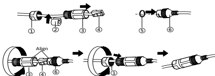
Рисунок 2-9 Установка гермоввода
