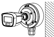
Рисунок 2-8 Установка крышки монтажной коробки на основание
