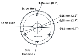
Рисунок 2-2 Шаблон крепления
