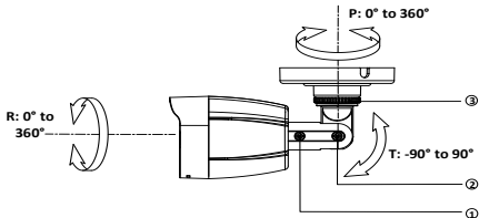
Рисунок 2-4 3-х осевая регулировка
