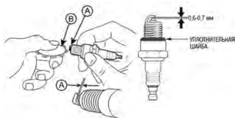
Рис. 13 Проверка зазора между электродами А – зазор, В – щуп
