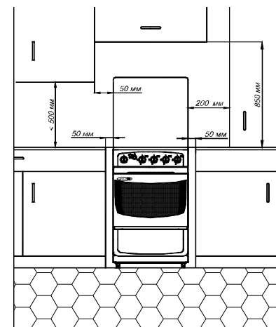
Рисунок 6 – Схема установки плиты
