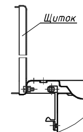
Рисунок 7 – Крепление щитка
