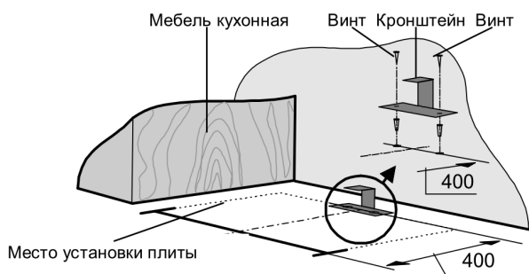
Рисунок 8 – Порядок установки кронштейна
