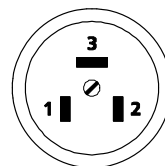
Рисунок 9 – Схема подключения розетки
