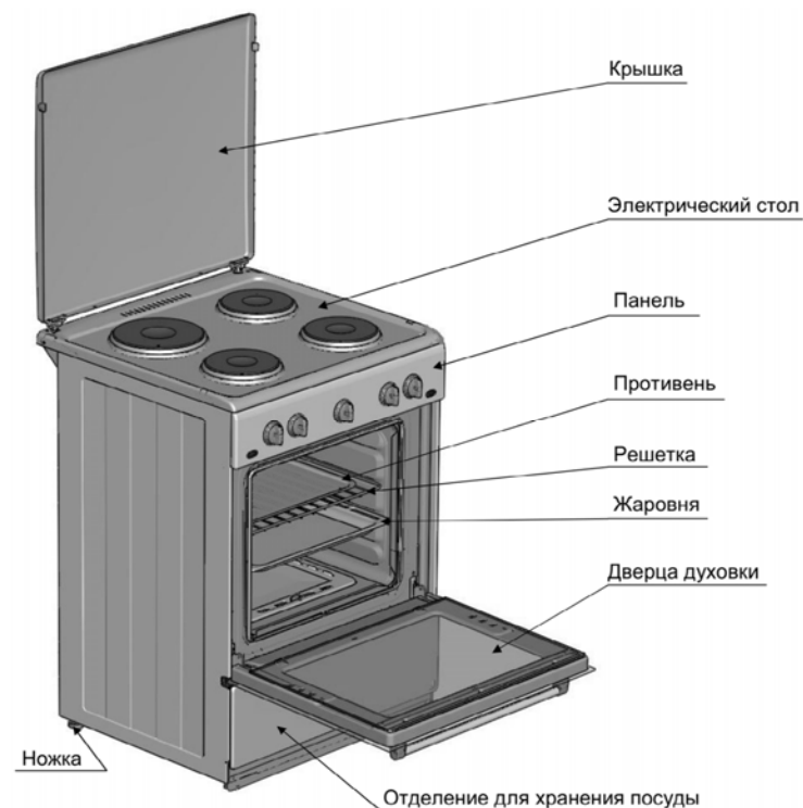
Рисунок 1 – Устройство плиты
