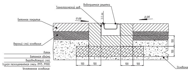
Схема монтажа водоотводного лотка Ecotek STANDART 100.95 H 99 в поверхность из бетонного покрытия. Класс нагрузки B 125 .
