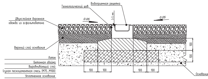
Схема монтажа водоотводного лотка Ecotek STANDART 100.95 H 99 в поверхность из асфальтобетонного покрытия. Класс нагрузки A 15 .
