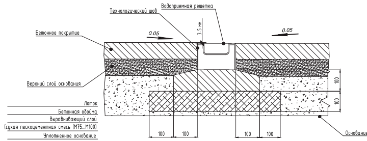
Схема монтажа водоотводного лотка Ecotek STANDART 100.95 H 99 в поверхность из бетонного покрытия. Класс нагрузки A 15 .
