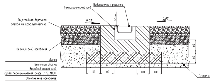
Схема монтажа водоотводного лотка Ecotek STANDART 100.95 H 99 в поверхность из асфальтобетонного покрытия. Класс нагрузки B 125 .
