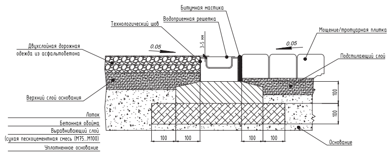
Схема монтажа водоотводного лотка Ecotek STANDART 100.95 H 99 в поверхность, мощеную штучным камнем и асфальтобетонным покрытием. Класс нагрузки A 15 .
