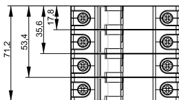
Рисунок 4 – Основные размеры
