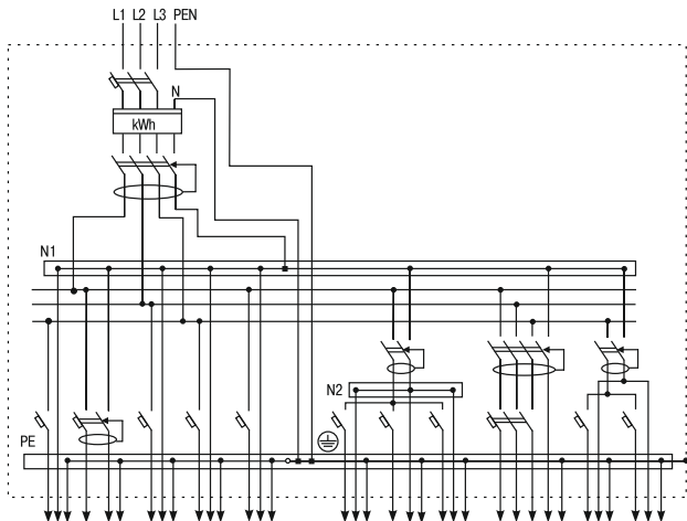
Рисунок 6 – Схема квартирного учетно-группового щитка (для коттеджа)
