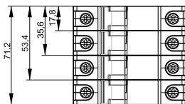
Рисунок 4 – Основные размеры
