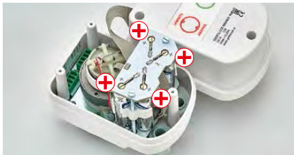
Фото 16. Электропривод со снятой верхней крышкой
