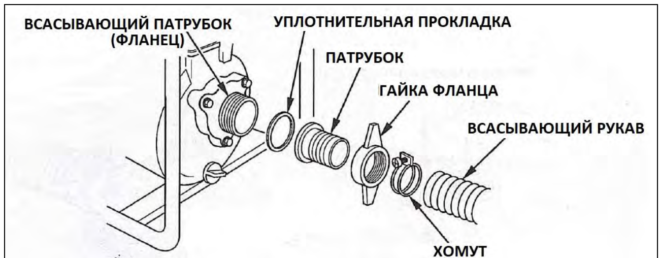
Рис.2 Порядок монтажа всасывающего рукава.
