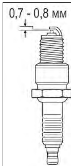
Рис. 17. Зазор свечи зажигания
