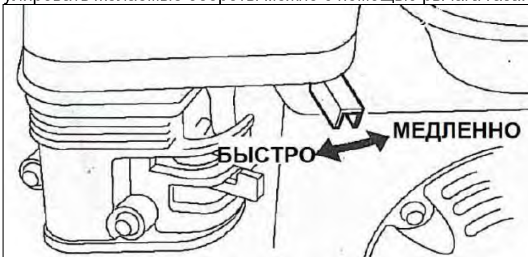
Рис. 12. Регулировка оборотов
