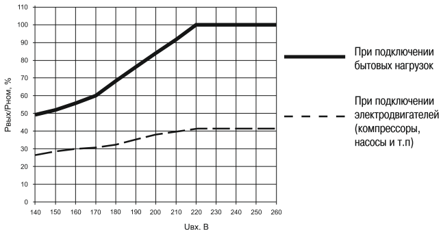
Рисунок 2 – Зависимость выходной мощности стабилизаторов от входного напряжения
