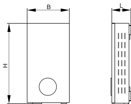
Рисунок 1 – Габаритные размеры стабилизаторов
