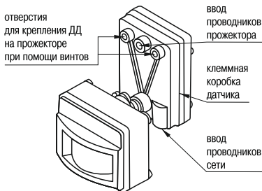
Рисунок 16 – Конструкция датчика движения ДД 017
