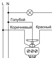
Рисунок 25 – Схема подключения датчика типа ДД 046
