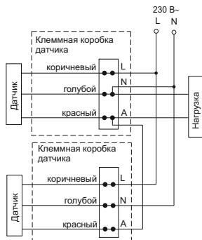
Рисунок 26 – Схема параллельного подключения датчиков
