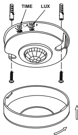
Рисунок 19 – Монтаж ДД 041
