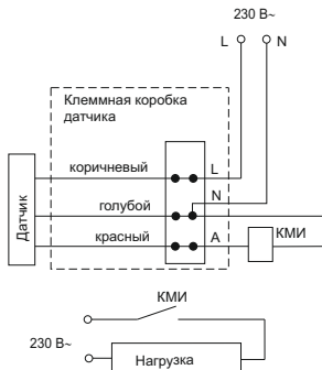
Рисунок 28 – Схема подключения датчика с контактором КМИ
