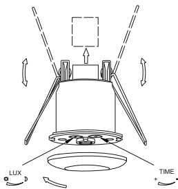
Рисунок 20 – Монтаж ДД 043
