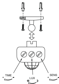
Рисунок 21 – Монтаж ДД 046
