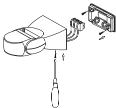
Рисунок 16 – Монтаж ДД 013
