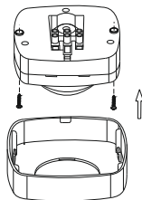
Рисунок 18 – Монтаж ДД 022, ДД 023
