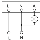
Рисунок 7 – Схема подключения датчика ДД 201
