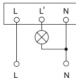
Рисунок 9 – Схема подключения датчика ДД 401
