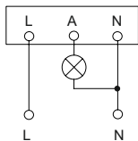
Рисунок 8 – Схема подключения датчика ДД 301
