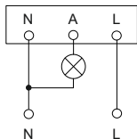
Рисунок 5 – Схема подключения датчика ДД 025, ДД 027
