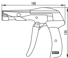
Рисунок 2 – ПКХ-600А
