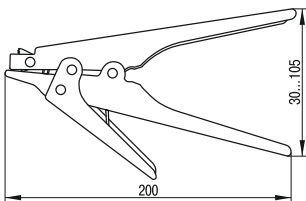
Рисунок 1 – ПКХ-519
