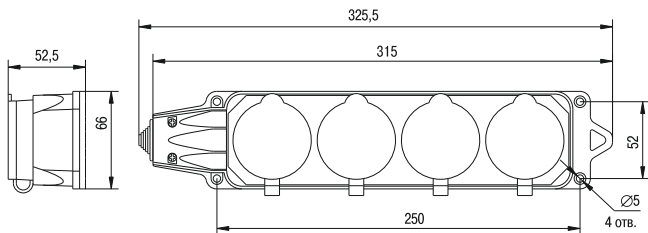
Рисунок 12 – Розетка (колодка) четырехместная с защитными крышками РБ34-1-0м
