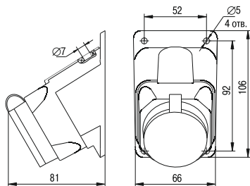
Рисунок 13 – Розетка с защитной крышкой угловая настенная РБу13-1-0м
