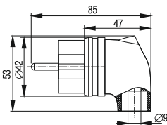
Рисунок 7 – Вилка с боковым вводом ВБу3-1-0м
