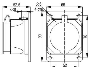
Рисунок 9 – Розетка с защитной крышкой настенная РБ13-1-0м
