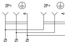
Рисунок 3 – Электрическая схема соединений РБЗ2-1-0м
