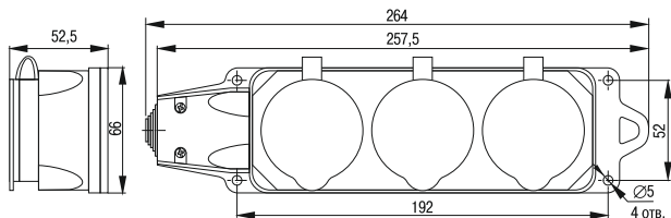
Рисунок 11 – Розетка (колодка) трёхместная с защитными крышками РБ33-1-0м
