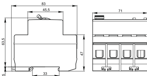
б) Четырехполюсные ВД
