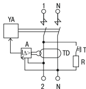
Рисунок 2 – Схема электрическая принципиальная двухполюсных ВД
