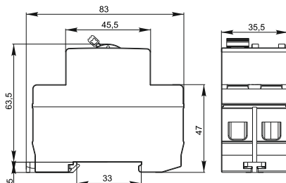
а) Двухполюсные ВД
