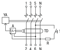
Рисунок 3 – Схема электрическая принципиальная четырехполюсных ВД
