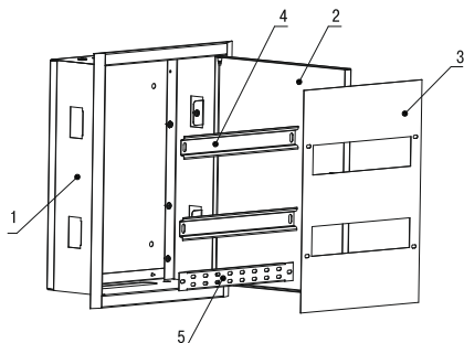
Рисунок 1 (1 – оболочка, 2 – дверь, 3 – панель, 4 – DIN-рейка, 5 – рейка)
