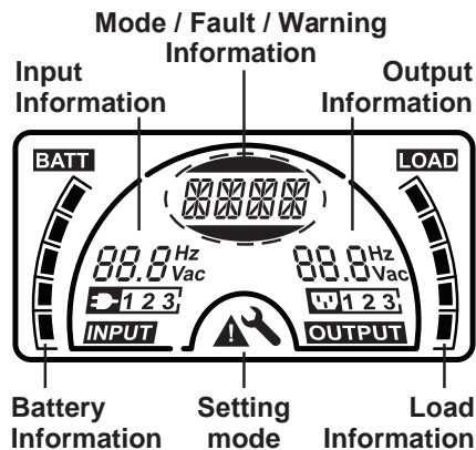
Рисунок 4.2 LCD дисплей
