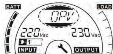
Рисунок 7.1 Настройки с помощью LCD-дисплея
