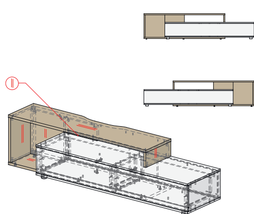
УНИВЕРСАЛЬНОЕ W3 / DI 1887 X 450 X 444
