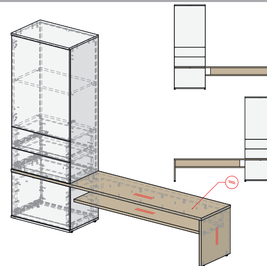
УНИВЕРСАЛЬНОЕ W3 / DI 1968 X 400 X 1632
