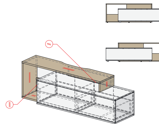
УНИВЕРСАЛЬНОЕ W3 / DI 1745 X 450 X 566
