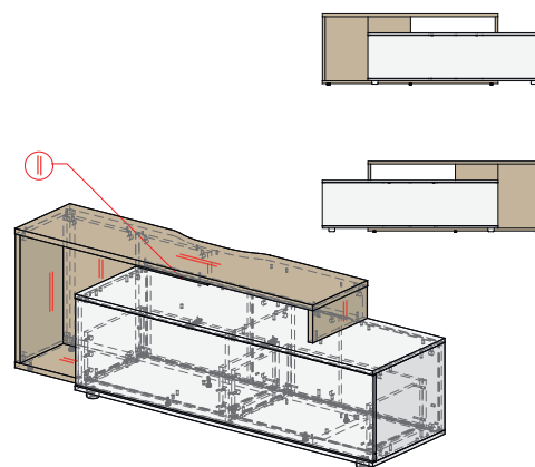
УНИВЕРСАЛЬНОЕ W3 / DI 1745 X 450 X 566
