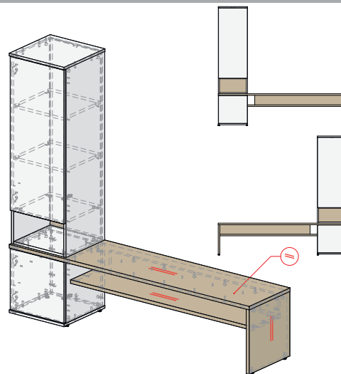
УНИВЕРСАЛЬНОЕ W3 / DI 1770 X 400 X 1632
