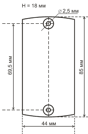
Рис.1 Габаритные размеры считывателя
