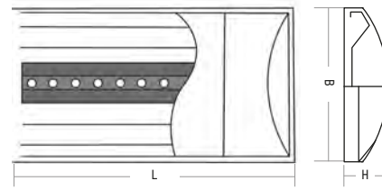
Рис. 1 Светильники PPO-03 600 / PPO-03 1200
