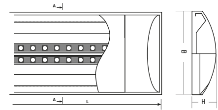
Рис. 2 Светильники PPO-03 1500
