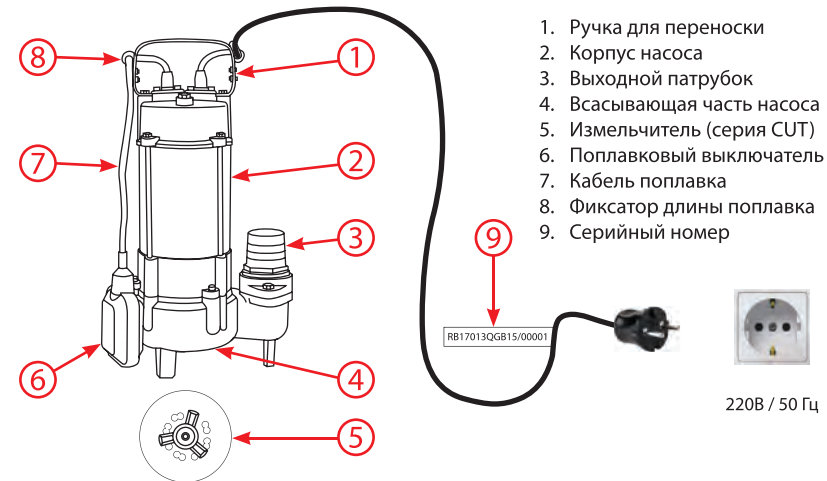
вид снизу (серия CUT)
