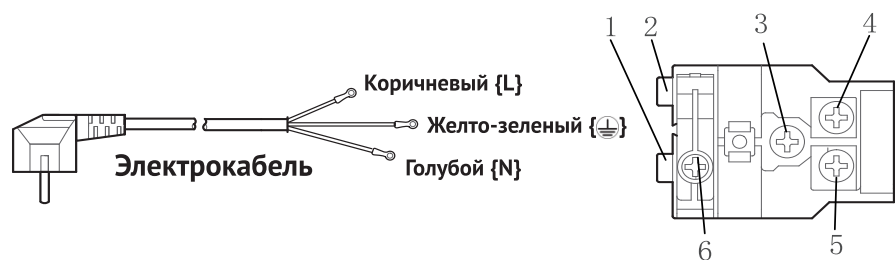
КЛЕММНАЯ КОРОБКА
