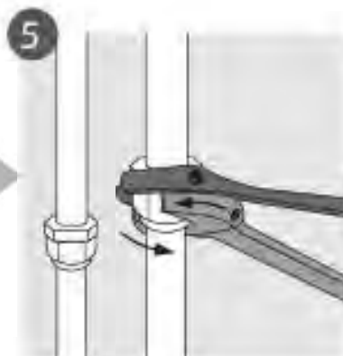
5 Подсоедините трубку
