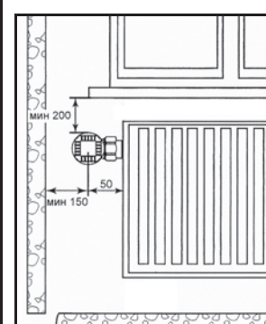
Рис. 5.4. Размещение терморегулятора
