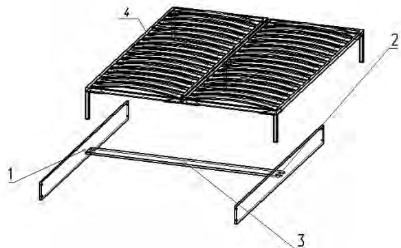
Рис.1 Схема сборки
