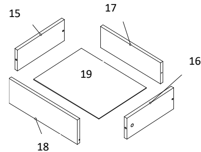
Рис.4 Схема сборки
