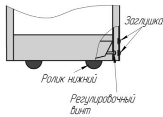
Рис.2 Схема регулировки
