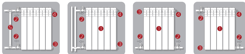
Диагональное (рекомендуется для получения максимальной теплоотдачи)
