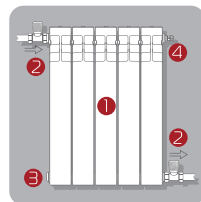
Диагональное (рекомендуется для получения максимальной теплоотдачи)
