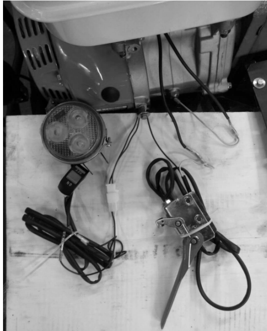
Схема подключения света (для моделей, оснащенных передней фарой)
