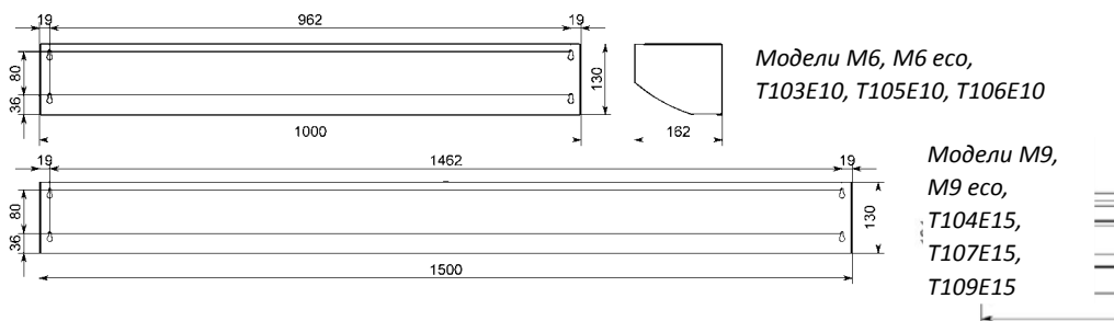
Рис. 2. Габаритные и установочные размеры приборов (Установка кронштейнов - опционально)
