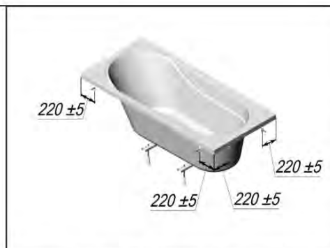
Рисунок 4- Схема расположения креплений кронштейнов к стене
