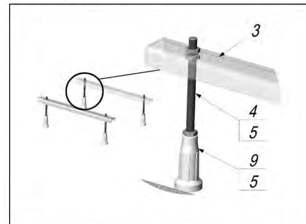
Рисунок 1- Сборка элементов каркаса ванны
