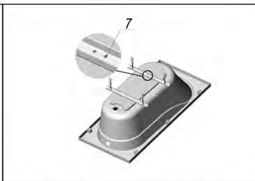
Рисунок 3- Фиксация каркаса ванны
