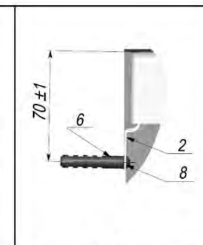
Рисунок 5- Крепление ванны к стене
