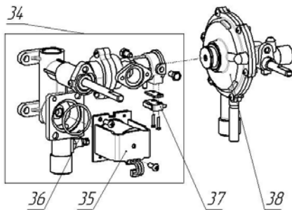
Рисунок 9. Узел водогазовый
