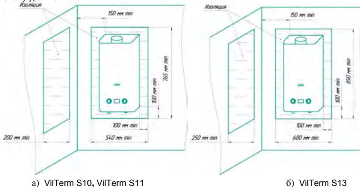
Рисунок 2. Пример установки аппаратов на труднодоступных стенах
