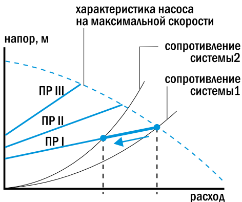
Рис.11 График работы насоса в режиме ПР.
