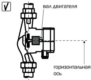
Рис.4 Установка циркуляционного насоса.
