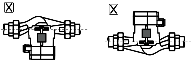
Рис.4.1 Неправильная установка насоса.
