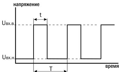
Рис.13 Характеристики ШИМ-сигнала.
