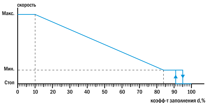
Рис.14 Зависимость скорости от коэффициента заполнения.
