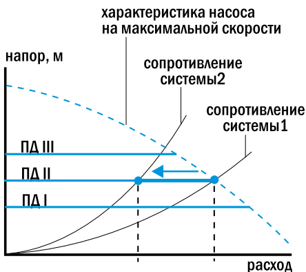
Рис.10 График работы насоса в режиме ПД.
