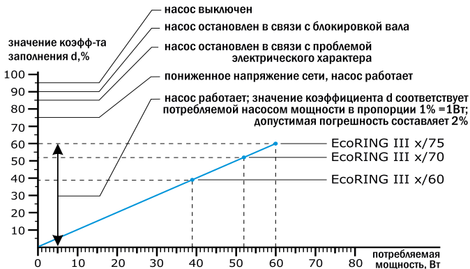
Рис.15 Зависимость коэффициента заполнения от состояния насоса.
