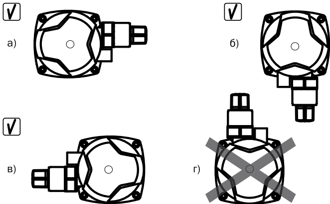
Рис.5 Правильное расположение насоса.
