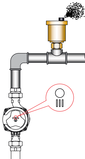
Рис.2 Удаление воздуха из корпуса насоса.
