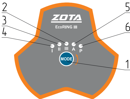
Рис.16 Органы управления.
