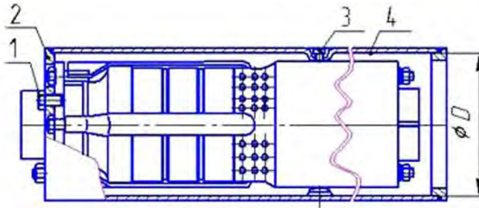
Рисунок 2. Кожух для больших диаметров скважины
