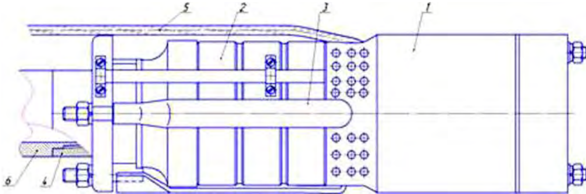
Рисунок 1. Устройство электронасосного агрегата.
