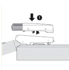
Монтаж демпфера
