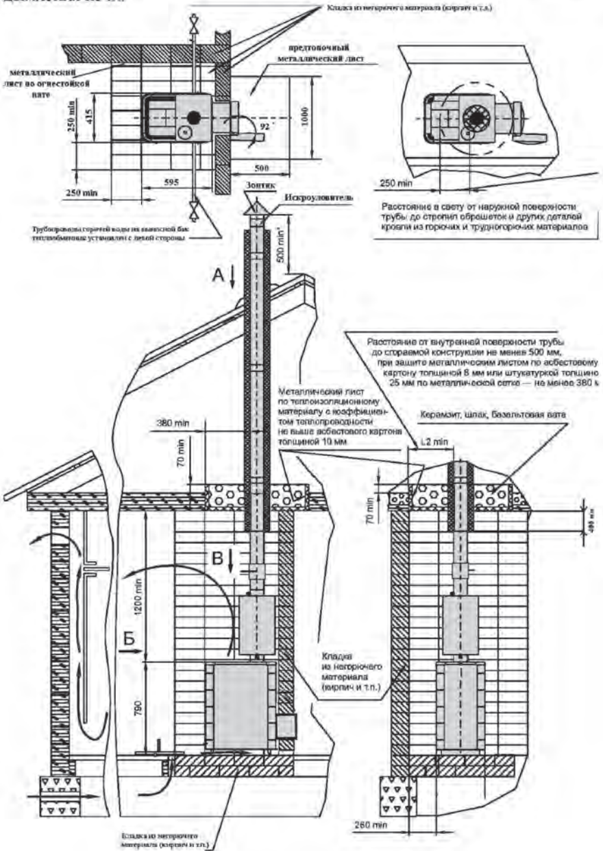
Схема монтажа печи
