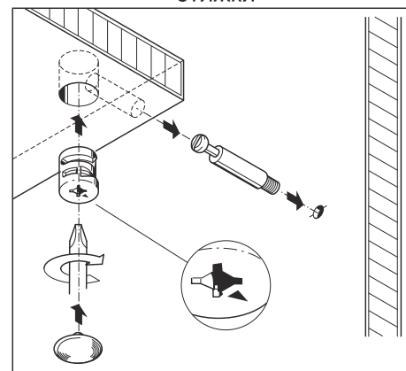
Монтаж эксцентрикостяжки
