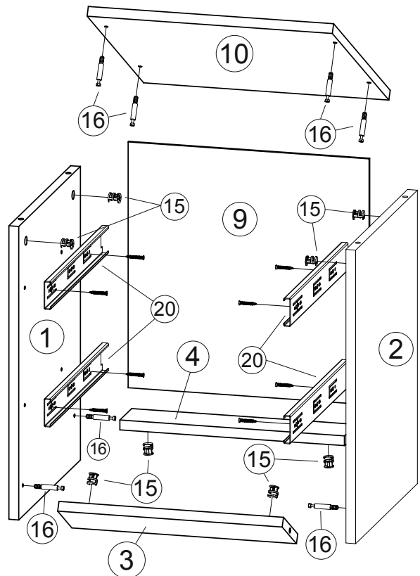
Рис.3 Сборка ящика
