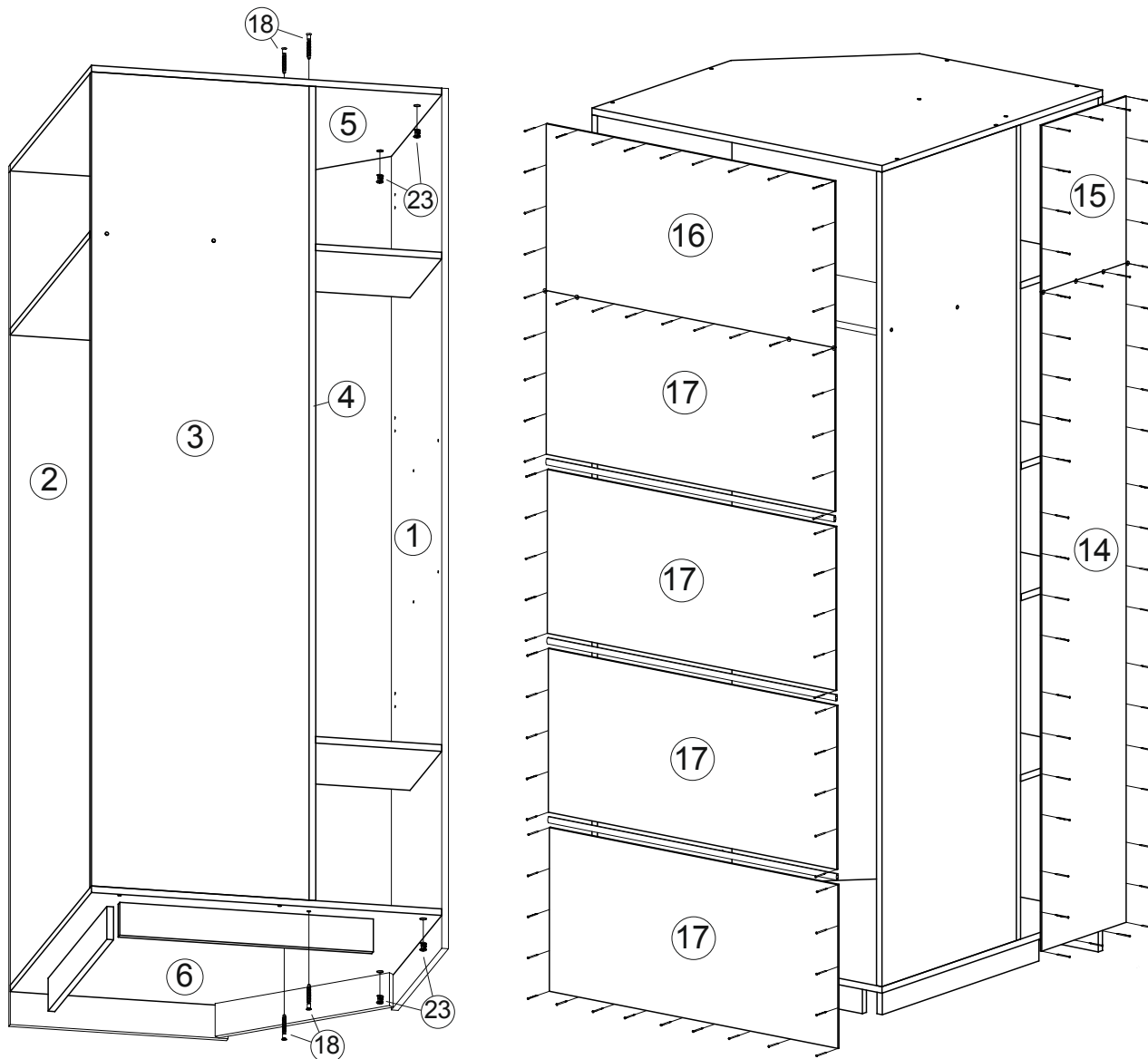
Рис.4 - Установка евровинта
