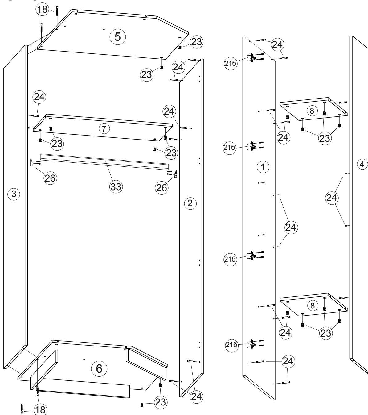
Рис.2 Сборка каркаса
