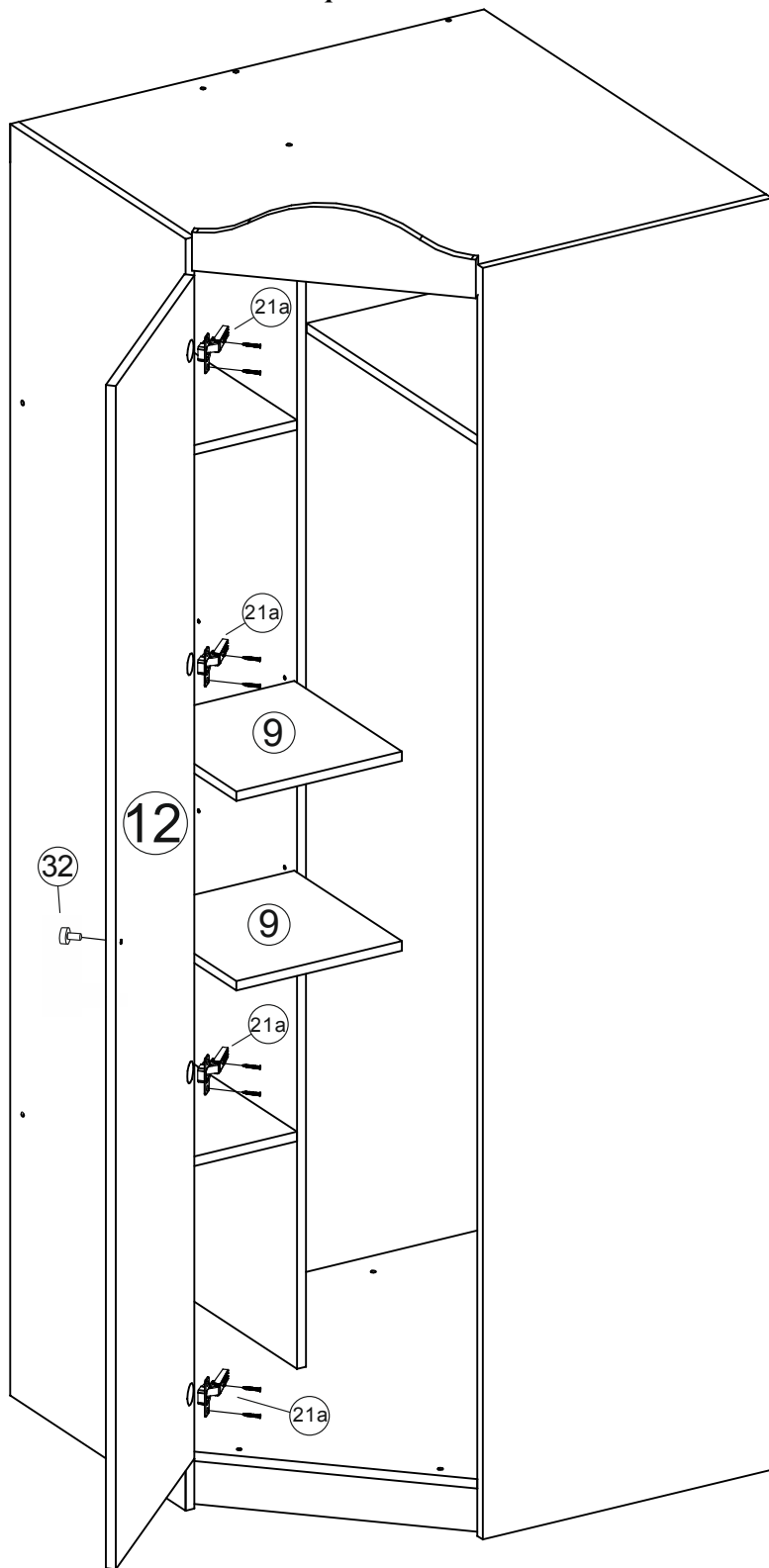
Рис.8 Окончательная сборка
