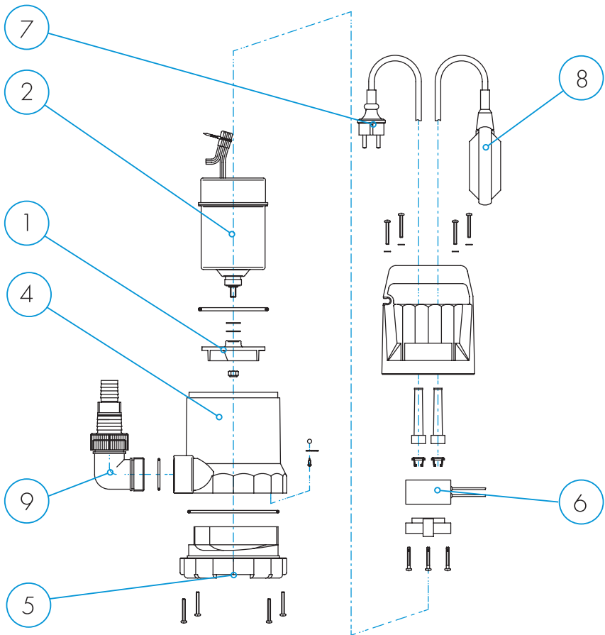
Рисунок 2 (на примере изображен насос погружной «ДРЕНАЖНИК» 110/6).
