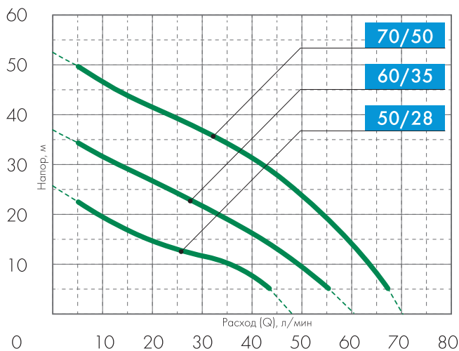
График расходно-напорных характеристик.
