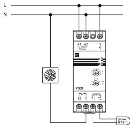
Рис. 3. Схема подключения
