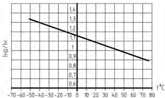
Рисунок А.3 - Зависимость номинального рабочего тока выключателей с приемкой РС от температуры окружающего воздуха
