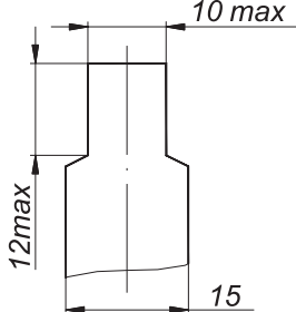
Рисунок 1 - Форма и размеры присоединяемой шины максимального сечения
