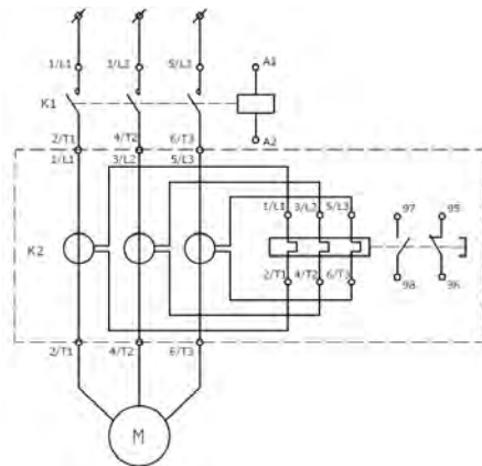
Рисунок Д.2 – Схема включения реле РТЛ-3000 и РТЛ-4000
