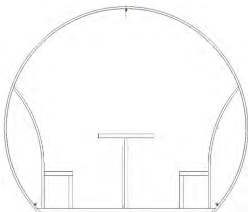
Схема №2 (а, б) – Соединение изогнутой стяжкой
