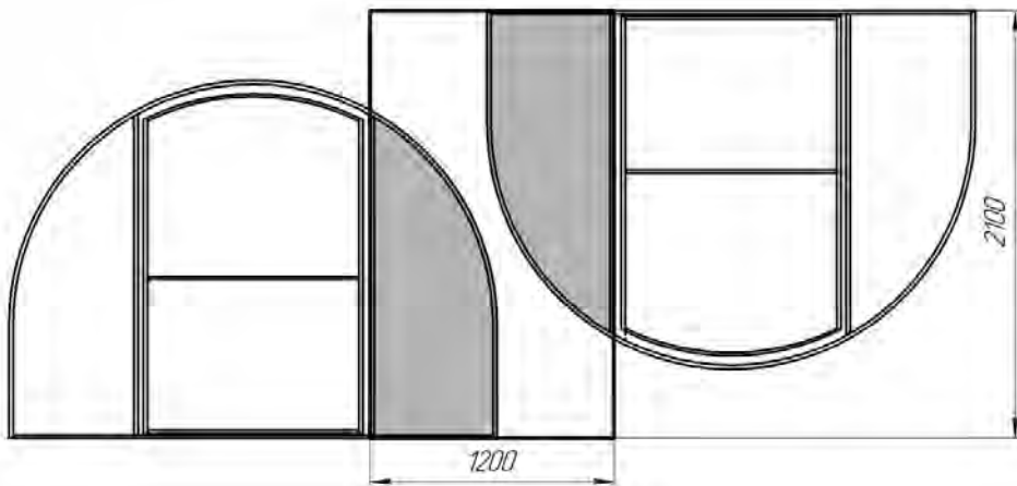
Рисунок 1 - Схема раскроя поликарбоната на торцы теплицы
