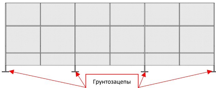
Рисунок 6 – Установка грунтозацепов
