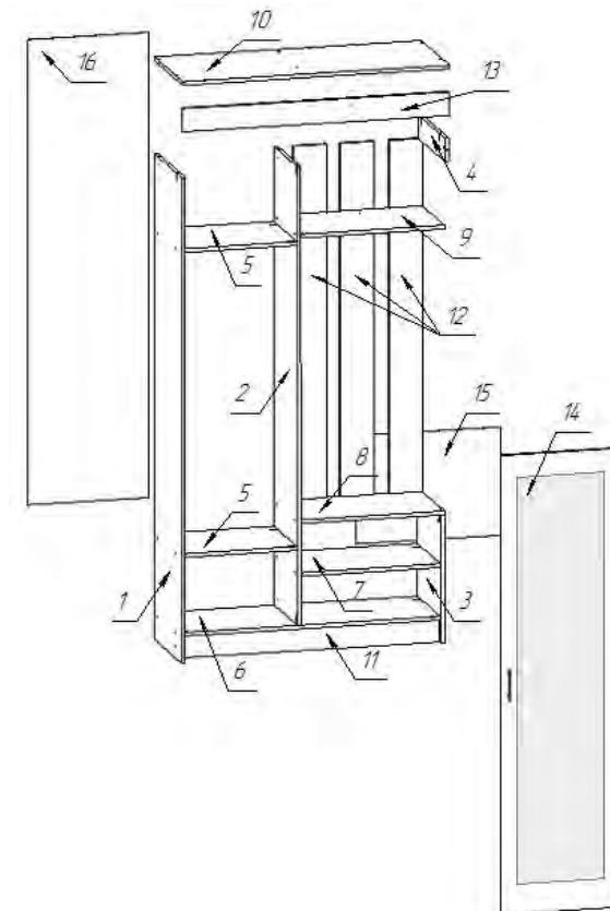
Взрыв-схема прихожей "ПВ-5":
