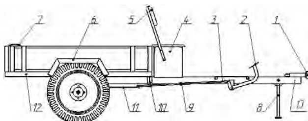
Рис.1 Тележка мотоблока
