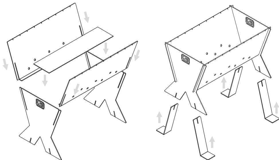
Рис. 2 Сборка мангала
